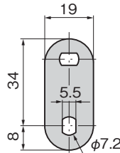
止め金 舌片
