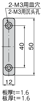
[C-74用受け金具] C-74用吸板
