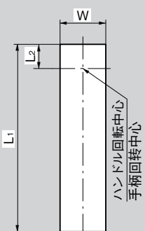
パネル穴明け寸法 面板开孔尺寸
