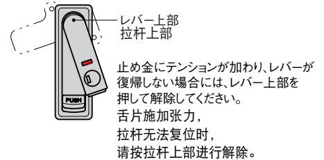
レバー復帰困難時の解除方法 拉杆复位困难时的解除方法
