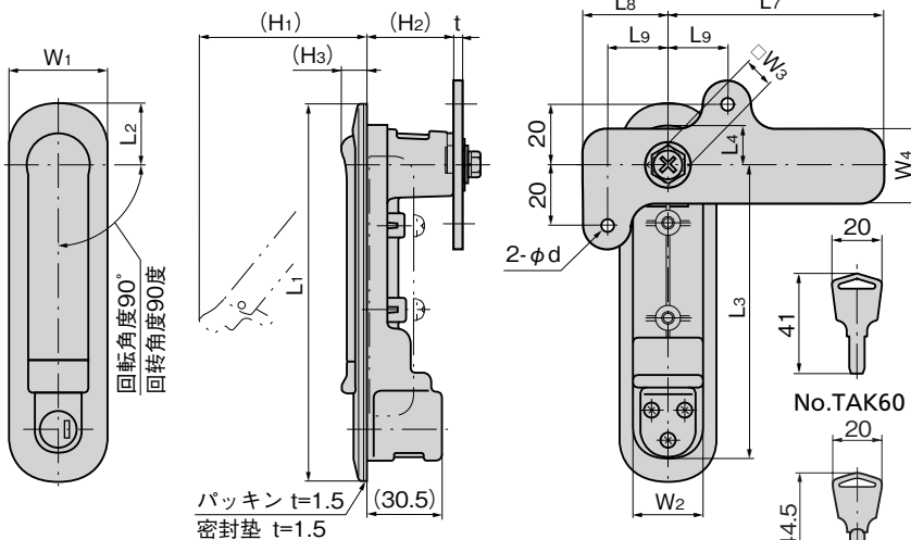
A-488-S-1
